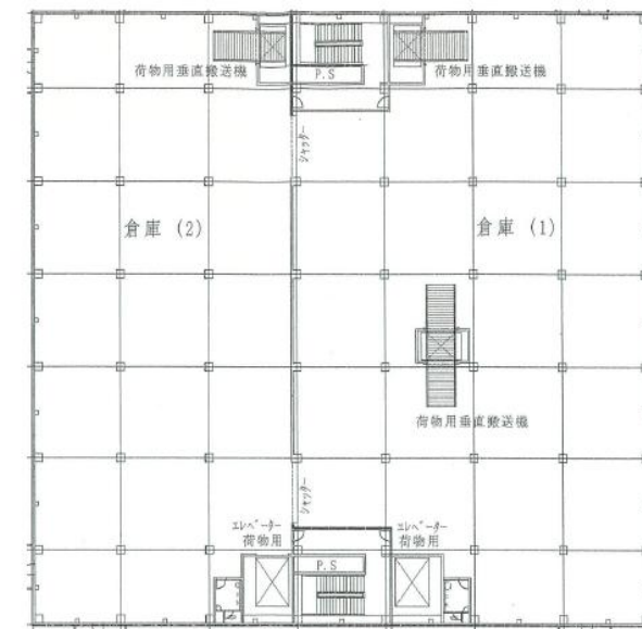
1階平面図
